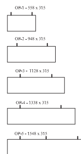
Oslony biurek z plyty 18mm :
