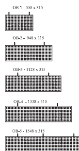
Oslony biurek z blachy perforowanej ;
