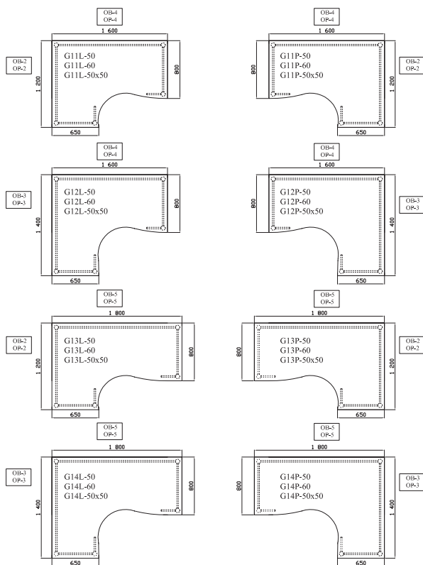
Oslony biurek z blachy perforowanej ;
