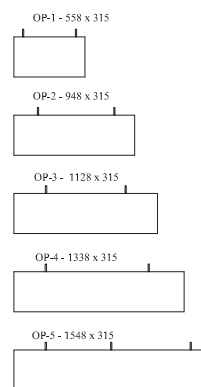
Oslony biurek z plyty 18mm :
