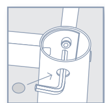
SPOSÓB ŁĄCZENIA BELEK Z NOGĄ
